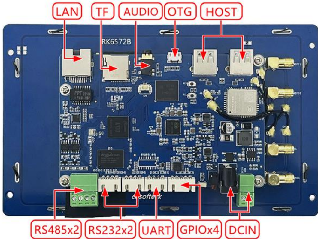
背面视图
